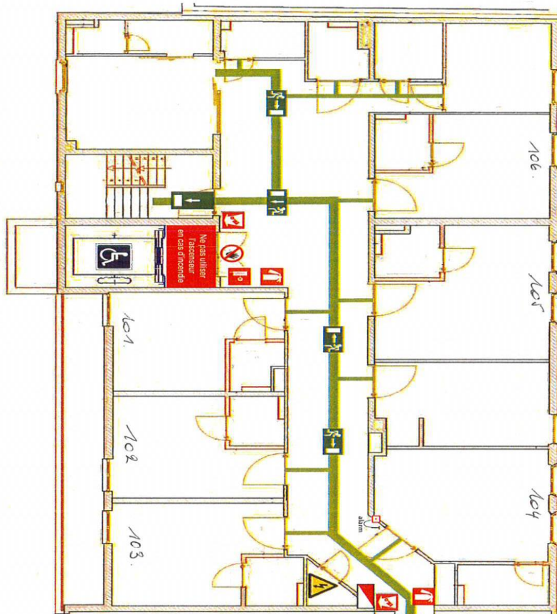
PLAN D'EVACUATION INCENDIE SERVICE SOINS PALLIATIFS - PREMIER ETAGE
